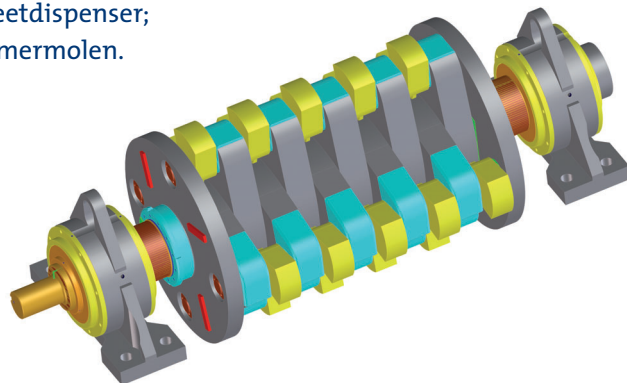
3D ontwerp hamermolen
